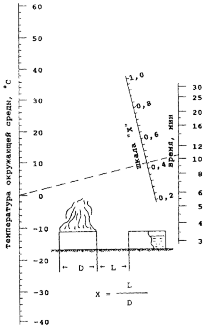
Рис. 1. Номограмма для определения максимально допустимого времени ввода сил и средств для охлаждения резервуаров, расположенных рядом с горящим
