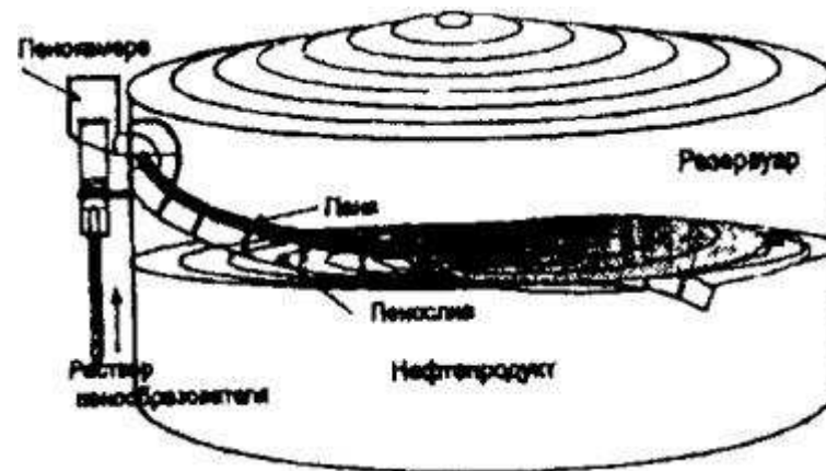
Рис. 2. Применение раздвижных пеносливов для плавной подачи пены на поверхность нефтепродукта
