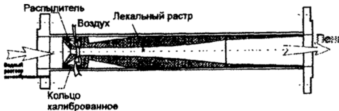
Рис. 2.2. Схема внутреннего устройства пеногенератора
