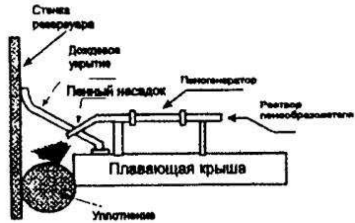
Рис. 8. Расположение пеногенирующей аппаратуры на плавающей крыше
