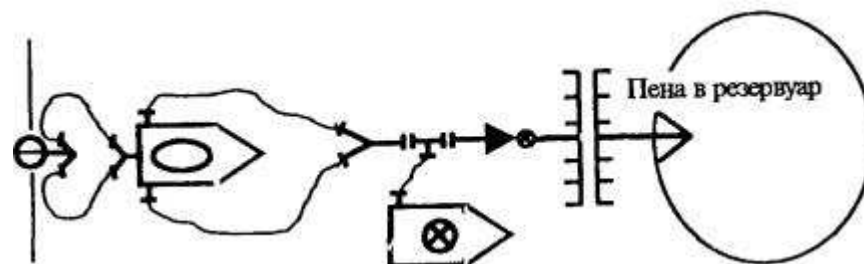
Рис. 2. Принципиальная схема подачи пены низкой кратности при тушении пожара в резервуаре подслоинным методом
